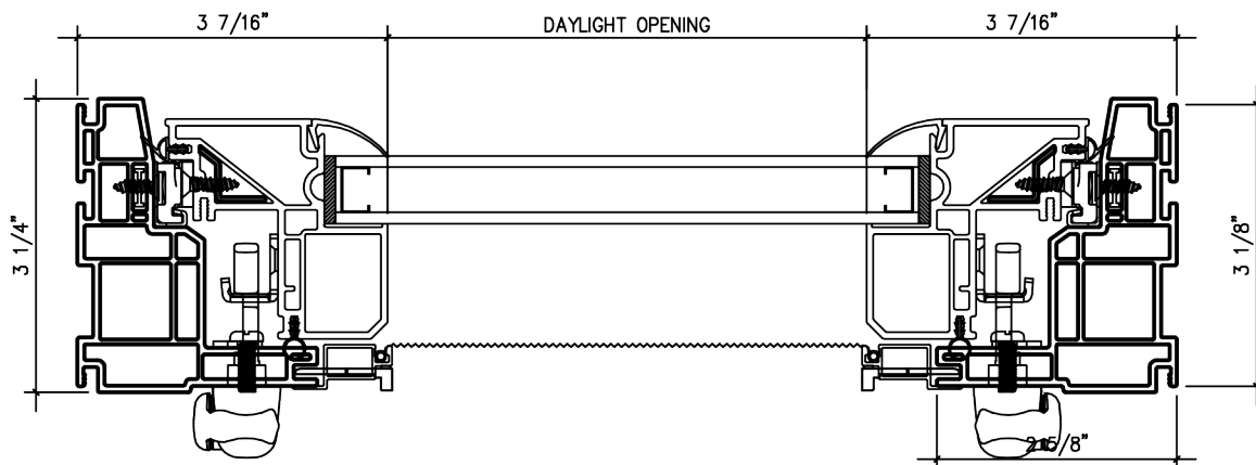
① Jamb Detail
